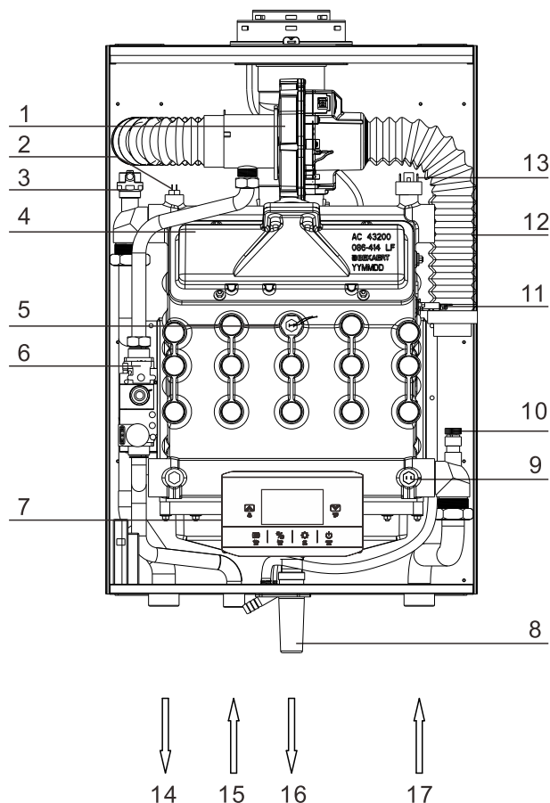
冷凝机结构示意图
